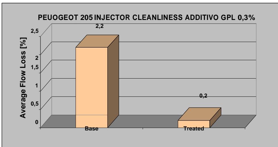
Grafico 3: benefici nell'utilizzo di ADDITIVO GPL in relazione alla perdita di flusso in aspirazione
