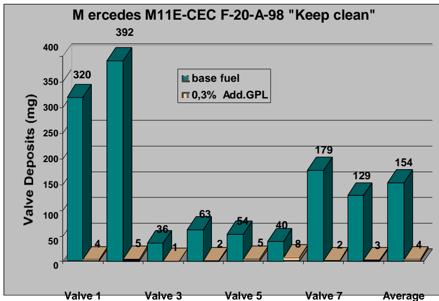
Grafico 5: benefici nell'utilizzo di PULITORE GPL in relazione ai depositi sulle valvole
