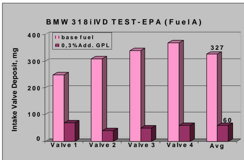
Grafico 6: benefici nell'utilizzo di PULITORE GPL in relazione ai depositi sulle valvole
