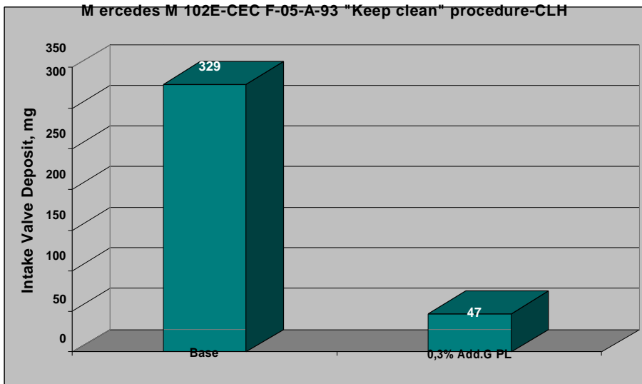
Grafico 2: benefici nell'utilizzo di ADDITIVO GPL in relazione ai depositi sulla valvola di aspirazione
