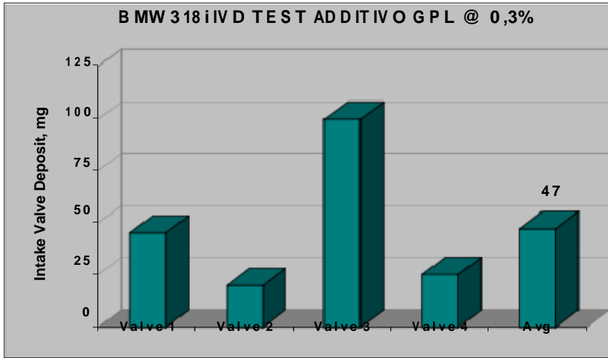
Grafico 1: depositi formatisi sulla valvola di aspirazione
