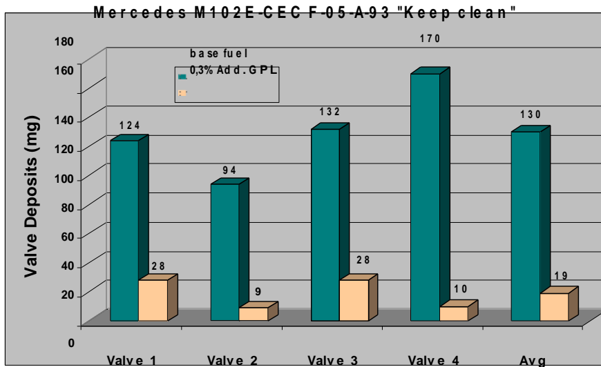
Grafico 4: benefici nell'utilizzo di PULITORE GPL in relazione ai depositi sulle valvole
